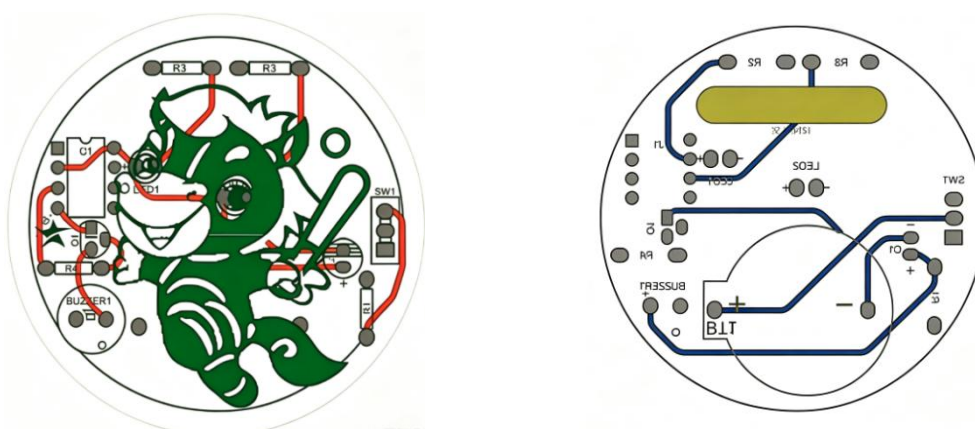
小学二、三年级及初中组趣味电子徽章 PCB 正反面
